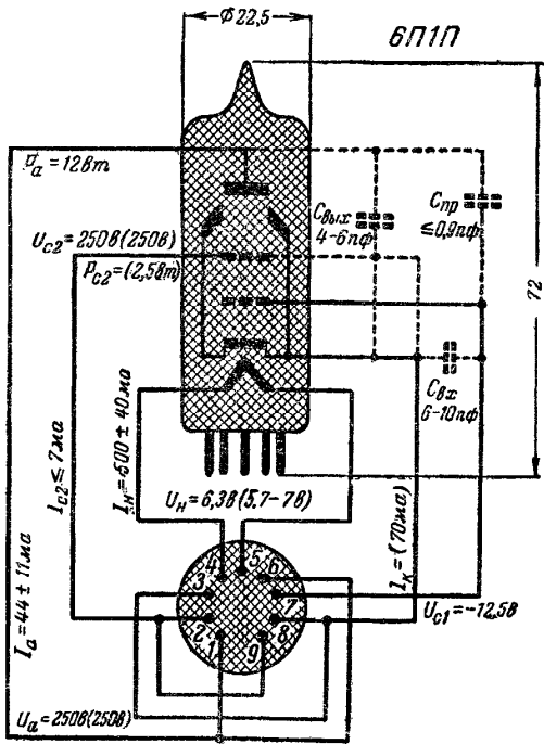
Рис. 13. Габаритный чертёж и схема соединений электродов с выводами тетрода 6П1П.
