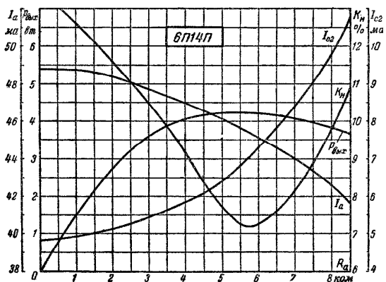
Рис. 33. Динамические характеристики выходной мощности P_{\text{вых}} , коэффициента нелинейных искажений K_H , тока анода I_a и тока сетки второй I_{c2} лампы 6П14П в зависимости от сопротивления анодной нагрузки R_a при U_a = U_{c2} = 250 в, R_K = 120 ом и \sim U_{c1} = 3,4 в (эфф.).
