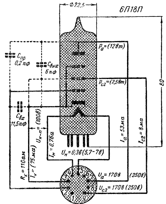
Рис. 37. Габаритный чертеж и схема соединений электродов с выводами пентода 6П18П.
