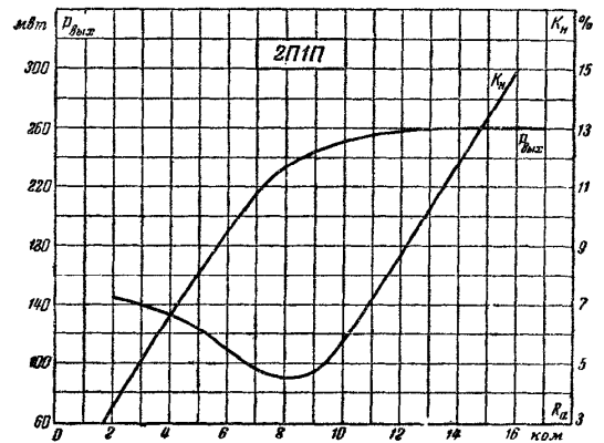
Рис. 5. Динамические характеристики выходной мощности P_{\text{вых}} и коэффициента нелинейных искажений K_n лампы 2П1П в зависимости от сопротивления анодной нагрузки R_a при U_a = U_{c2} = 90 \text{ в} , U_{c1} = -4,5 \text{ в} и \sim U_{c1} = 3,2 \text{ в} (эфф.)
