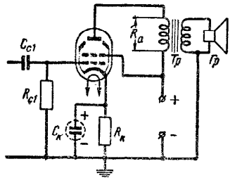
Рис. 1. Схема оконечного каскада усиления низкой частоты.
