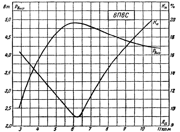
Рис. 25. Динамические характеристики выходной мощности P_{\text{вых}} и коэффициента нелинейных искажений K_{\text{н}} лампы 6П6С в зависимости от сопротивления анодной нагрузки R_a при U_a = U_{c2} = 250 в, U_{c1} = -12,5 в и \sim U_{c1} = 8,8 в (эфф.).
