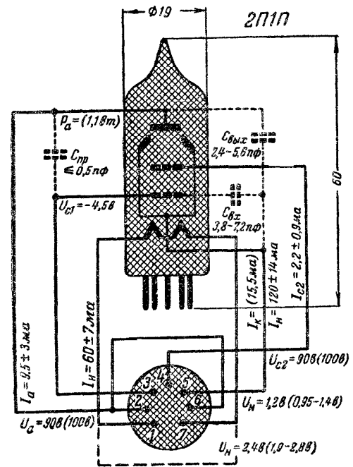
Рис. 2. Габаритный чертеж и схема соединений электродов с выводами тетрода 2П1П.
