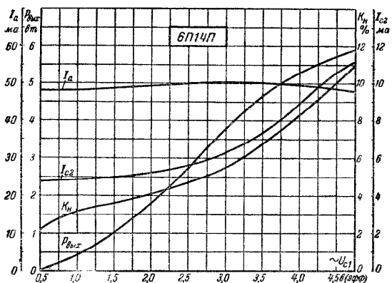
Рис. 32. Динамические характеристики выходной мощности P_{\text{вых}} , коэффициента нелинейных искажений K_H , тока анода I_a и тока сетки второй I_{c2} лампы 6П14П в зависимости от эффективного напряжения сетки первой \sim U_{c1} при U_a = U_{c2} = 250 в, U_{c1} = -6 в и R_a = 5 к.ом.
