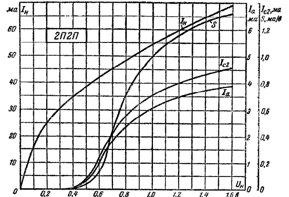
Рис. 7. Характеристики тока анода I_a , тока сетки второй I_{c2} , крутизны S и тока накала I_n лампы 2П2П в зависимости от напряжения накала U_n при U_a = U_{c2} = 60 в и U_{c1} = -3,5 в.
