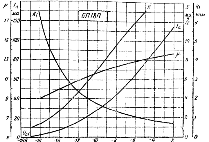
Рис. 44. Анодно-сеточная I_a , крутизна S , коэффициента усиления \mu и внутреннего сопротивления R_i характеристики лампы 6П18П в триодном включении (анод соединен с сеткой второй) при U_a = 170 в.
