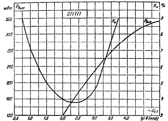
Рис. 4. Динамические характеристики выходной мощности P_{\text{вых}} и коэффициента нелинейных искажений K_n лампы 2П1П в зависимости от эффективного напряжения сетки первой \sim U_{c1} при U_a = U_{c2} = 90 \text{ в} , U_{c1} = -4,5 \text{ в} и R_a = 10 \text{ ком} .
