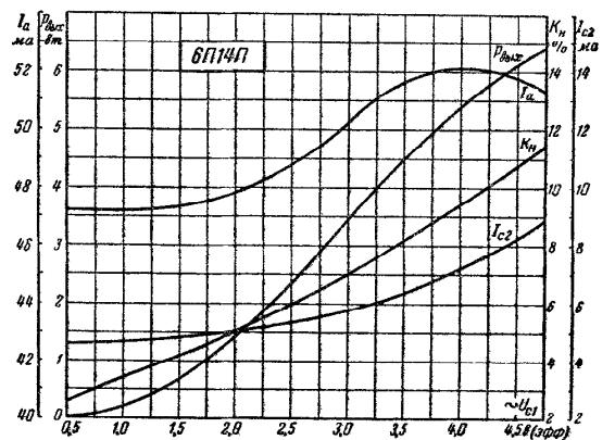
Рис. 31. Динамические характеристики выходной мощности P_{\text{вых}} , коэффициента нелинейных искажений K_n , тока анода I_a и тока сетки второй I_{c2} лампы 6П14П в зависимости от эффективного напряжения сетки первой \sim U_{c1} при U_a = U_{c2} = 250 в, U_{c1} = -6 в и R_a = 4 ком.
