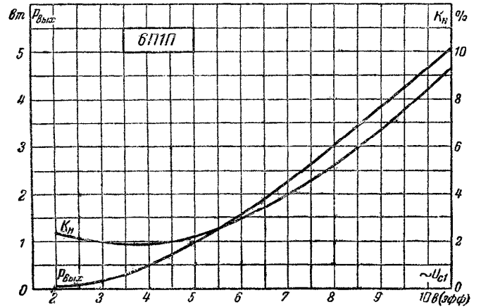
Рис. 15. Динамические характеристики выходной мощности P_{\text{вых}} и коэффициента нелинейных искажений K_N лампы 6П1П в зависимости от эффективного напряжения сетки первой U_{c1} при U_a = U_{c2} = 250 в, U_{c1} = -12,5 в R_a = 5 ком.
