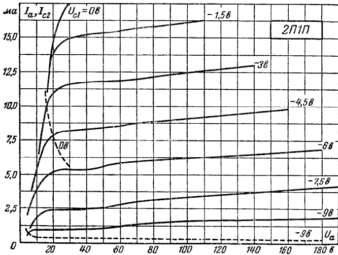
Рис. 3. Анодные (сплошные) и сеточно-анодные по сетке второй (штриховые) характеристики лампы 2П1П при U_{c2} = 90 \text{ в} .
