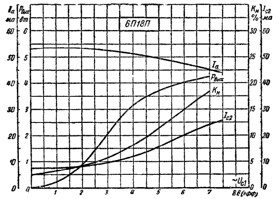
Рис. 41. Динамические характеристики выходной мощности P_{\text{вых}} , коэффициента нелинейных искажений K_n , тока анода I_a и тока сетки второй I_{c2} лампы 6П18П в зависимости от эффективного напряжения сетки первой \sim U_{c1} при U_a = U_{c2} = 177 в, R_n = 110 ом и R_a = 3 ком.
