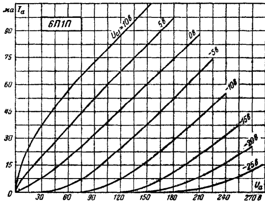
Рис. 17. Анодные характеристики лампы 6П1П в триодном включении (анод соединен с сеткой второй).
