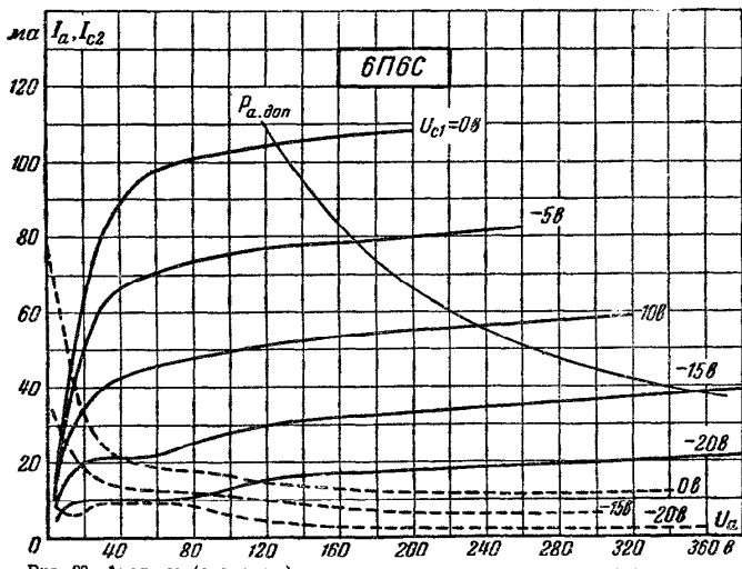
Рис. 23. Анодные (сплошные) и сеточно-анодные по сетке второй (штриховые) характеристики лампы 6П6С при U_{c2} = 250 в.
