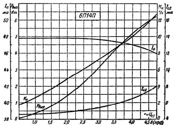
Рис. 35. Динамические характеристики выходной мощности P_{\text{вых}} , коэффициента нелинейных искажений K_H , тока анода I_a и тока сетки второй I_{c2} лампы 6П14П в зависимости от эффективного напряжения сетки первой \sim U_{c1} при U_a = U_{c2} = 256 в, R_K = 120 ом и R_a = 4 к.ом.
