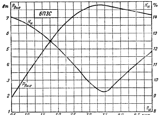
Рис. 21. Динамические характеристики выходной мощности P_{\text{вых}} и коэффициента нелинейных искажений K_n лампы 6П3С в зависимости от сопротивления анодной нагрузки R_a при U_a = U_{c2} = 250 в, U_{c1} = -14 в и \sim U_{c1} = 9,8 в (эфф.).
