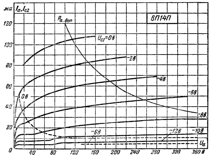
Рис. 27. Анодные (сплошные) и сеточно-анодные по сетке второй (штриховые) характеристики лампы 6П14П при U_{c2} = 250 v .
