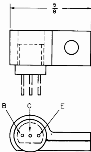
⑦ TO-98/w FLAG
