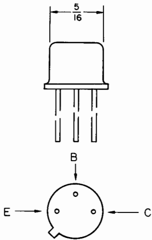
① TO-5 & TO-39
