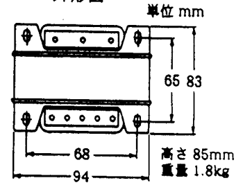
外形図
